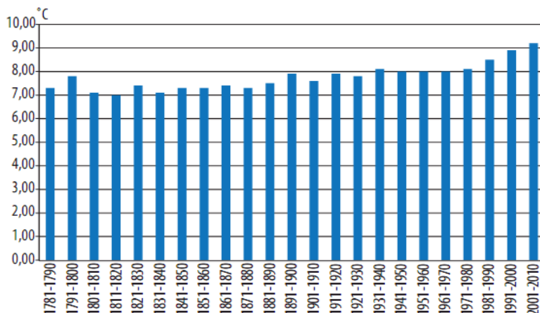
Ryc. 1. Wartości średniej rocznej temperatury powietrza w dziesięcioleciu na podstawie pomiarów stacji meteorologicznej Warszawa – Obserwatorium w latach 1791–2010 [źródło: Stan środowiska w Polsce – Raport 2014, GIOŚ 2014 za IMGW-PIB].
