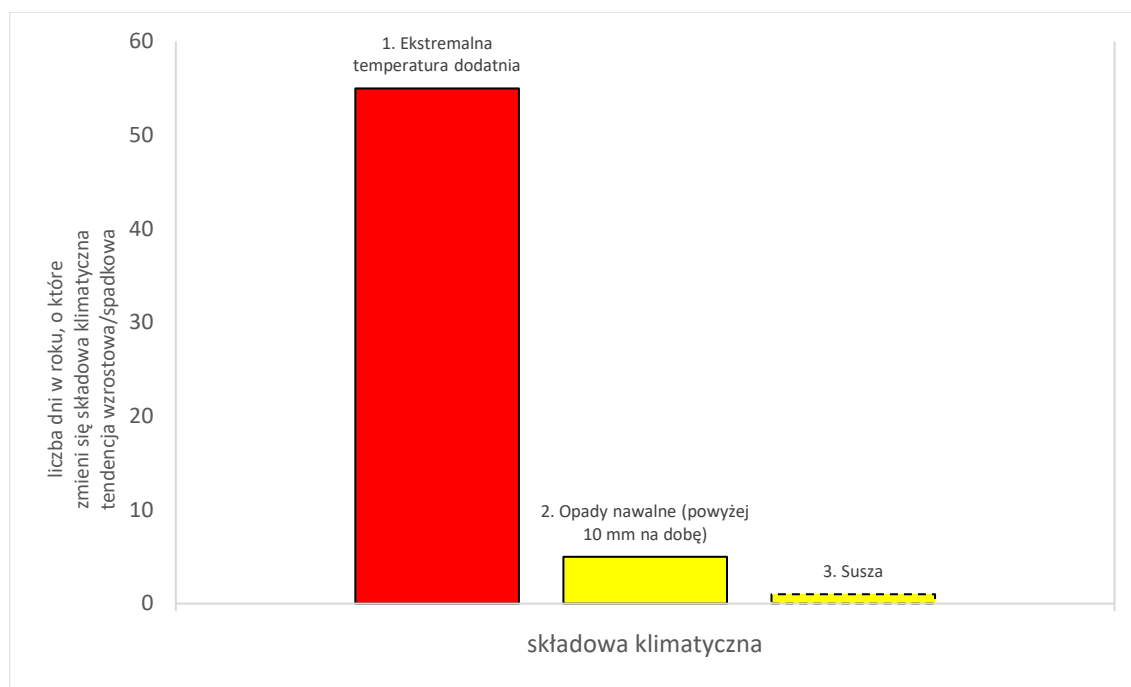
Wykres 4-1. Prognozowane tendencje zmian wybranych składowych klimatu.
