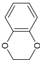
etylenodioksyferyl-
