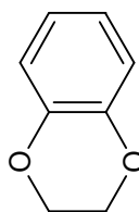
etylenodiodoksyfenyl-
