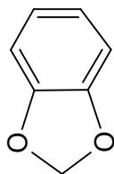
metylenodioksyferyl-
