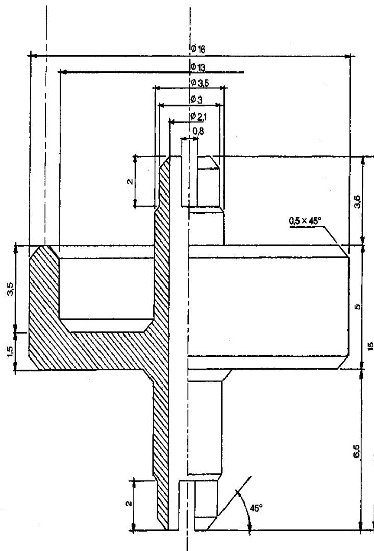
Rys. 1 Łącznik P1
