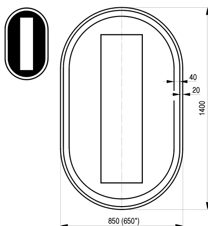
Rys. 10.29. Ekran kontrastowy owalny dla sygnalizatorów o soczewkach Ø 300 zawieszanych nad jezdnią * – dla sygnalizatorów o soczewkach Ø 300 umieszczanych obok jezdni
