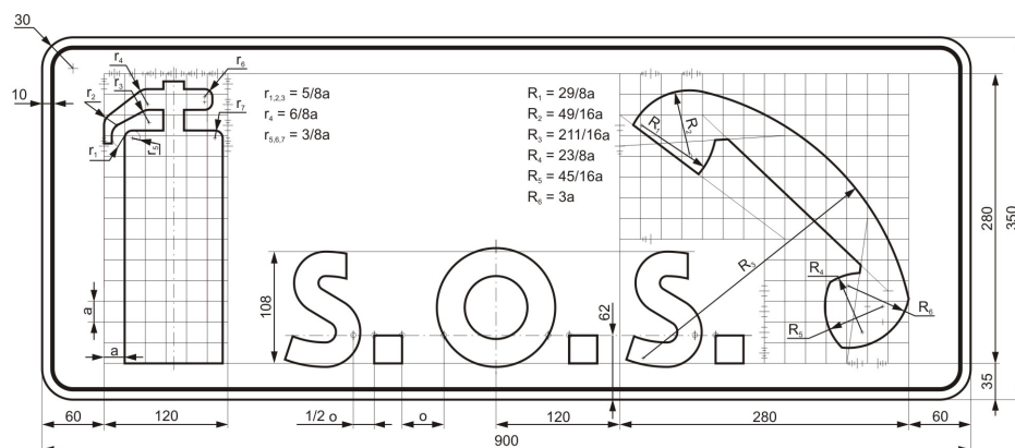
Rys. 9.7.53. Konstrukcja tabliczki T-33”;
