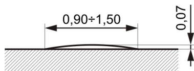
Rys. 8.1.4. Liniowy próg zwalniający listkowy U-16d o ograniczonej prędkości przejazdu 18–20 km/h
