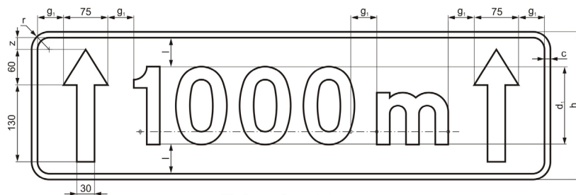
Rys. 9.7.1a. Konstrukcja tabliczki T-1b,
