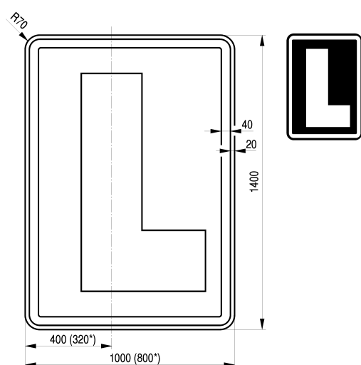
Rys. 10.30. Ekran kontrastowy prostokątny dla sygnalizatorów S-2 o soczewkach Ø 300 umieszczanych nad jezdnią wraz z sygnałem dopuszczającym skręcanie w prawo (symetryczny układ dla sygnału dopuszczającego skręcanie w lewo) * – dla sygnalizatorów o soczewkach Ø 300 umieszczanych obok jezdni
