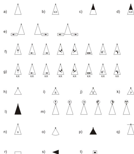
Rys. 7.1.3. Symbole graficzne sygnalizatorów i detektorów:
