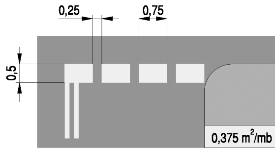
Rys. 4.2.5.1. Znak P-14
