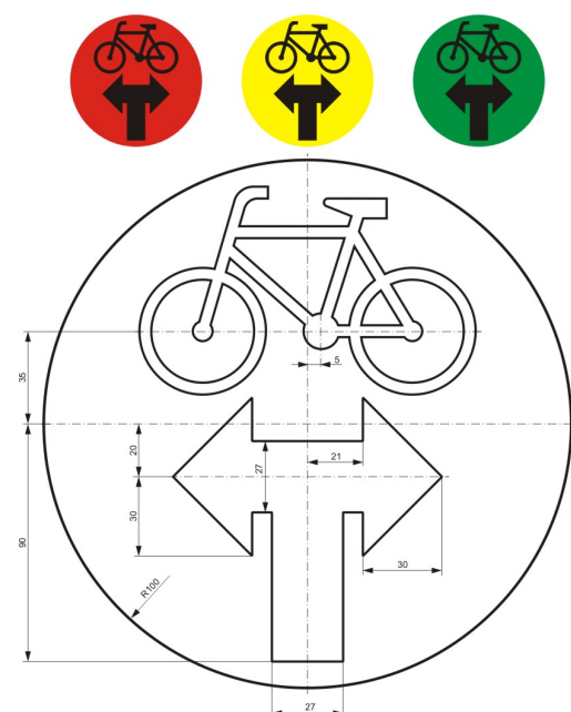
Rys. 10.9. Strzałki kierunku jazdy w prawo i w lewo na sygnalizatorze kierunkowym S-3a dla kierujących rowerem. Wymiary sylwetki roweru należy zmniejszyć do 75% wymiarów określonych na rysunku 10.1
