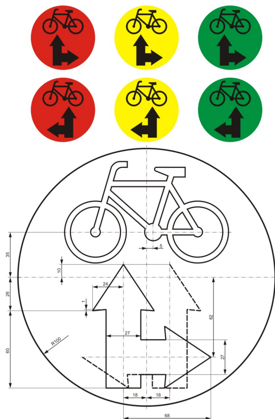
Rys. 10.6. Strzałki kierunku jazdy na wprost i w prawo lub na wprost i w lewo (odbicie zwierciadlane) na sygnalizatorze kierunkowym S-3a dla kierujących rowerem. Symbol strzałek na wprost i w lewo obrócony o 90° w lewo dotyczy jazdy w lewo i zawracania. Wymiary sylwetki roweru należy zmniejszyć do 75% wymiarów określonych na rysunku 10.1
