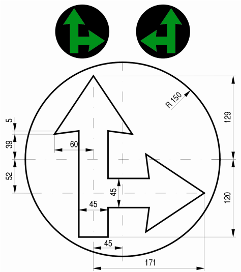
Rys. 10.4. Strzałki kierunku jazdy na wprost i w prawo lub na wprost i w lewo (odbicie zwierciadlane) dla sygnału zielonego. Symbol strzałek na wprost i w lewo obrócony o 90^\circ w lewo dotyczy jazdy w lewo i zwracania
