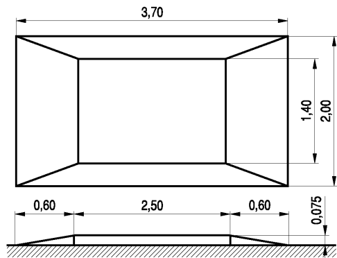
Rys. 8.1.6. Przykłady progów zwalniających wyspowych:
