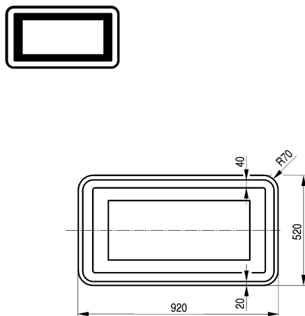
Rys. 10.32. Ekran kontrastowy dla sygnalizatorów S-4 z soczewkami Ø 300
