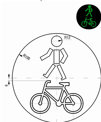
Rys. 10.21. Sylwetka roweru w sygnałach dla rowerzystów; przy średnicy \varnothing 100 ( \varnothing 90 ) wymiary należy zmniejszyć o 50%
