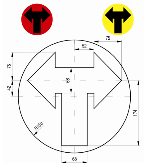
Rys. 10.8. Strzałki kierunku jazdy w prawo i w lewo dla sygnału czerwonego i żółtego
