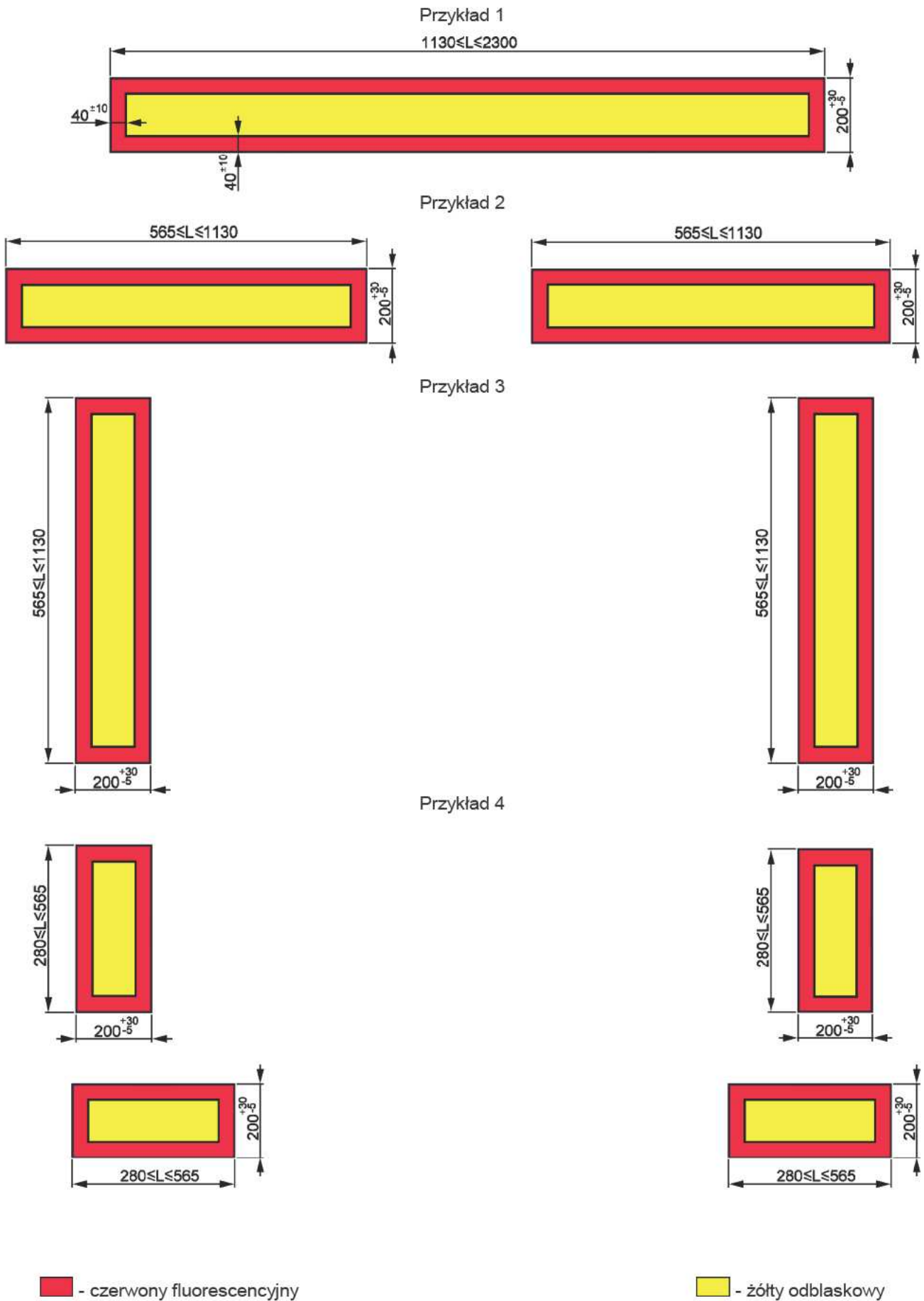
Rys. 2. Tablice wyróżniające przyczepę (naczepę) (mm)
