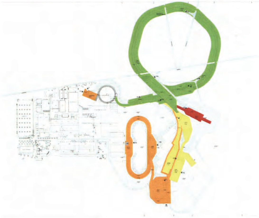
Rys 1: Modułowa Wersja Startowa FAIR. Kolory modułów: 0 – zielony; 1 – czerwony; 2 – żółty; 3 – pomarańczowy. Moduły 4 do 6 są zaznaczone bez kolorów. Nie jest zaznaczony dodatkowy eksperymentalny obszar na powierzchni, który jest częścią Modułu 1. Po lewej stronie rysunku jest pokazany istniejący ośrodek GSI.
