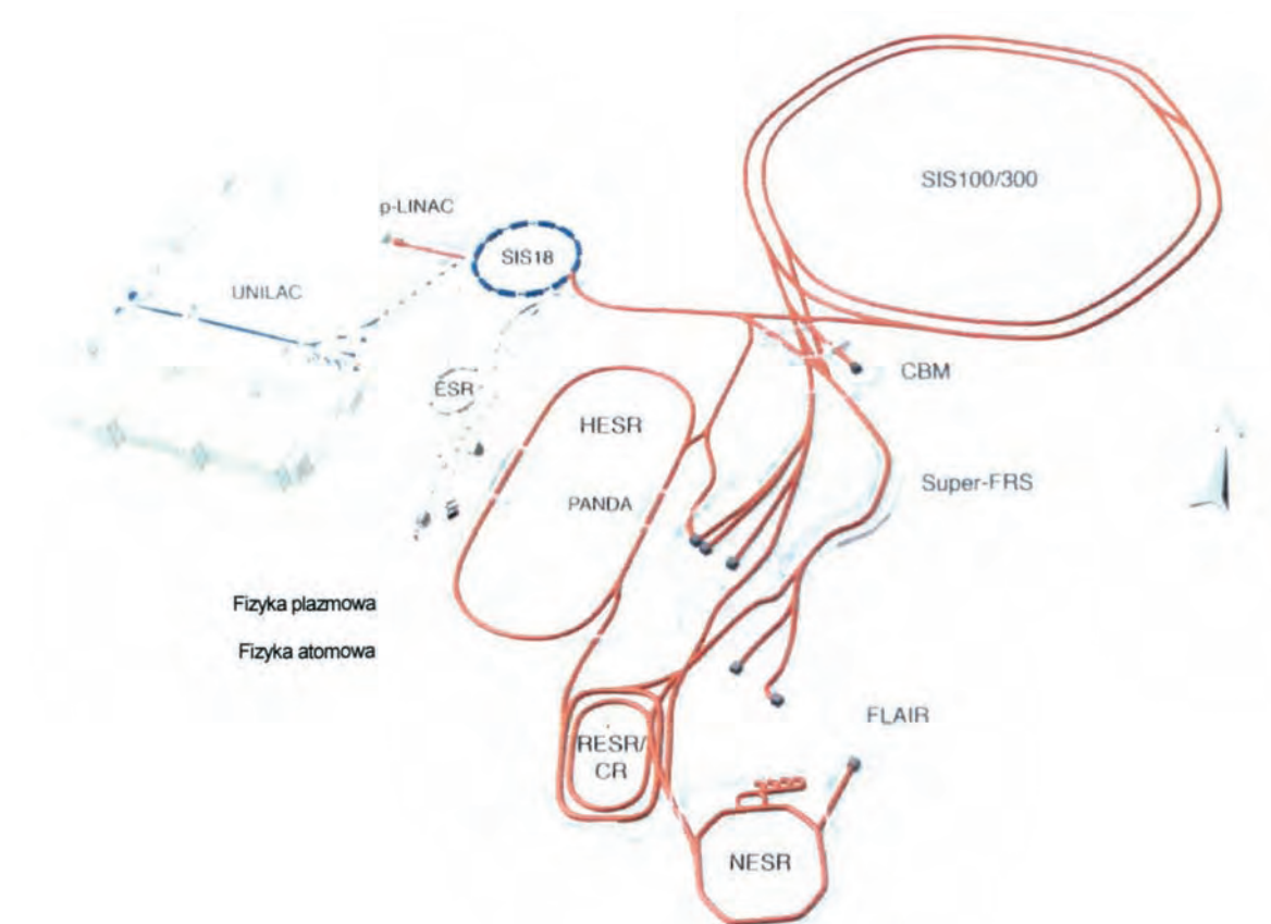
Rysunek 1: Rozkład przestrzenny Ośrodka FAIR: Akceleratory istniejące w GSI (niebieskie po lewej) funkcjonują jako akcelerator wstrzykujący dla nowych systemów akceleratorowych, które mają zostać zbudowane (czerwone po prawej).
