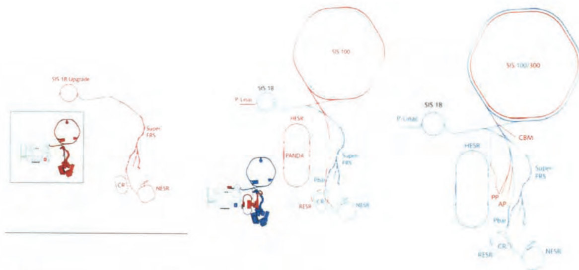
Rysunek 3: Fazy budowy i działania ośrodka FAIR. W pierwszej fazie (po lewej) zbudowane zostaną tylko elementy oznaczone na czerwono. Wstawka pokazuje działania z zakresu inżynierii lądowej wykonywane w fazie 1. W fazie drugiej (w środku) zbudowane zostaną elementy zaznaczone na czerwono, zaś elementy akceleratora zaznaczone na niebiesko będą już działały. Budynki oznaczone na niebiesko już będą istniały. W fazie trzeciej (po prawej) nie będą wykonywane prace z zakresu inżynierii lądowej. Budowane będą komponenty akceleratora oznaczone na czerwono.
